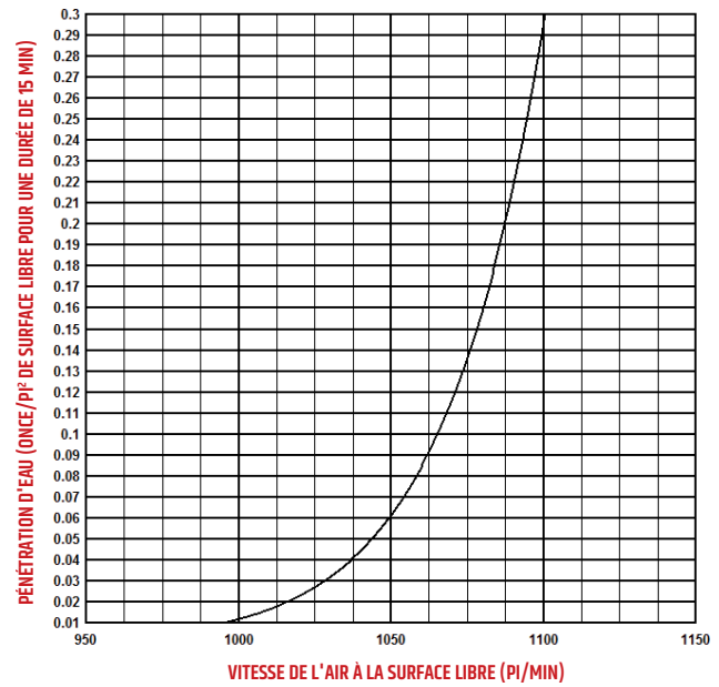
PÉNÉTRATION D'EAU MODÈLE ACOUSTIQUE 8" DÉBUT DE LA PÉNÉTRATION D'EAU À 996 PI/MIN
