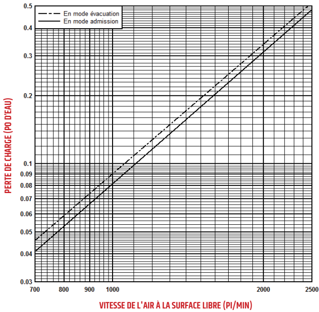
PERTE DE CHARGE VS VITESSE DE L'AIR MODÈLE ACOUSTIQUE 8"
